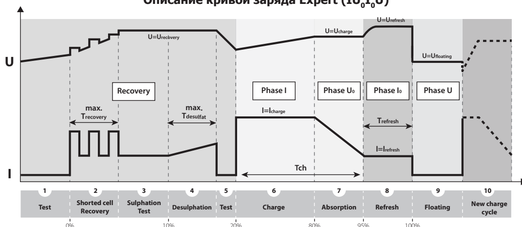
Описание кривой заряда Expert (I U , I 0 , U)
