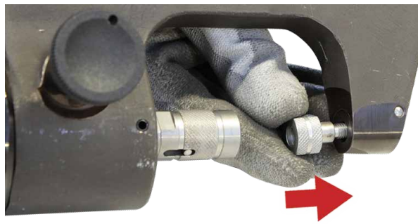
Matrice rivetto
