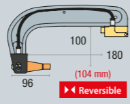
G1 8 bar/550 daN 022768
